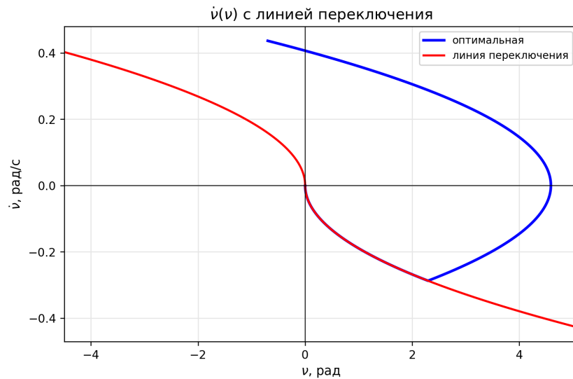
Рис. 5 – Фазовая траектория спутника при моделировании оптимального управления
