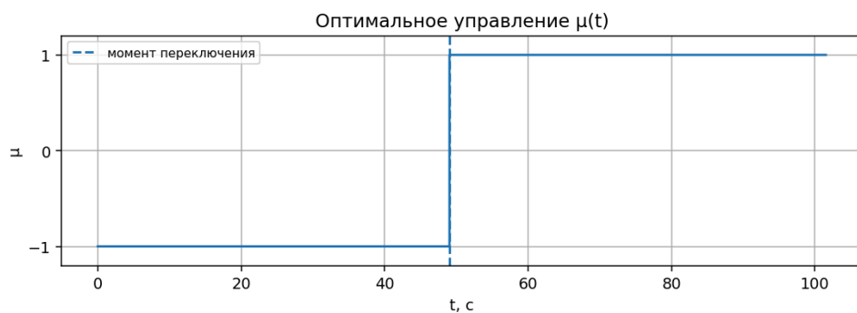
Рис. 12 – Закон оптимального управления \mu(t) для перехода спутника в точку (0.5; 0.5)
