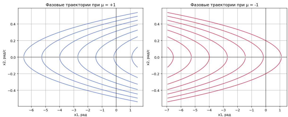
Рис. 9 – Фазовые траектории спутника при постоянных управлениях \mu = +1 и \mu = -1 для перехода в точку (0.5; 0.5)
