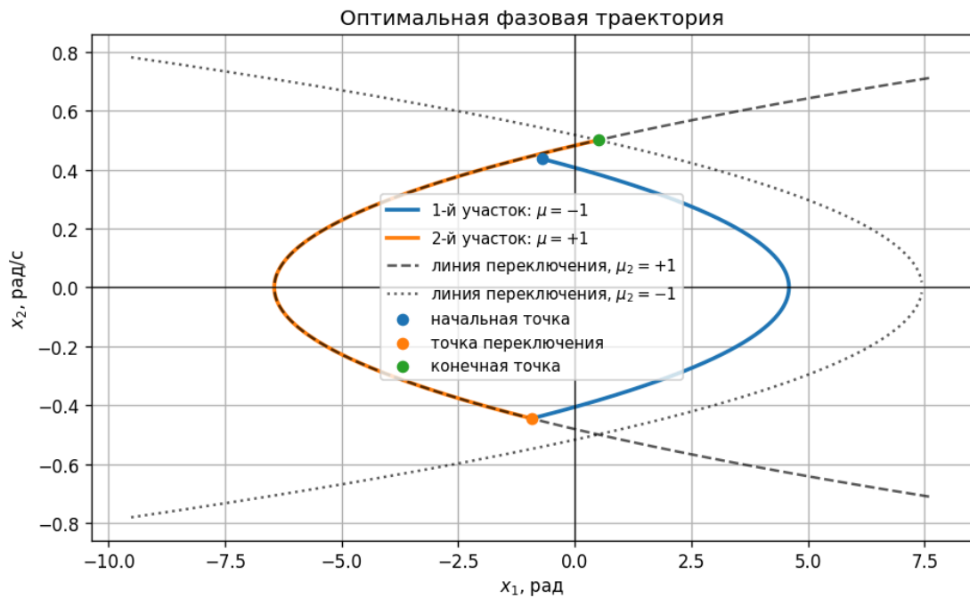
Рис. 10 – Оптимальная фазовая траектория перехода спутника в точку (0.5; 0.5)
