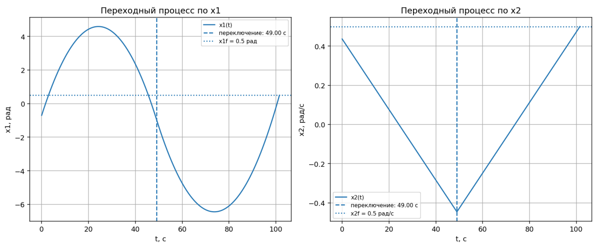
Рис. 11 – Переходные процессы x_1(t) и x_2(t) при переходе спутника в точку (0.5; 0.5)
